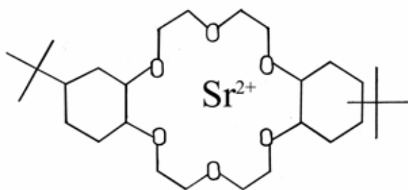
Рисунок 2 – Структурная формула краун-эфира 4,4'(5')-ди-{трет-бутил-циклогексан}-18-краун-6
