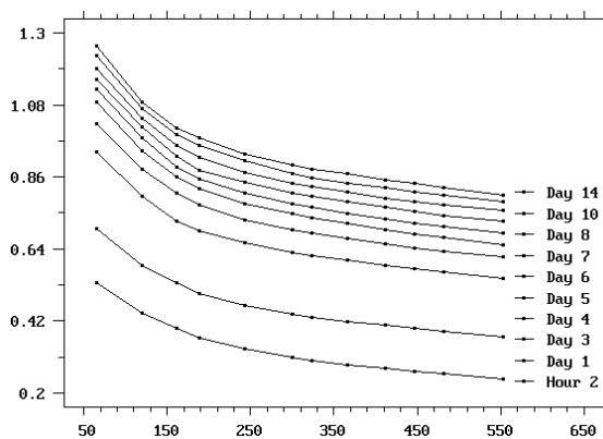
Рисунок 1 – Номограмма для определения коэффициента регистрации детектора в зависимости от массы осадка (мг) и времени накопления вторичного ^{90}\text{Y}
