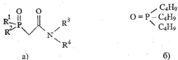
Рисунок 5 – Общая структура производных КМФО (а) и структура ТБФ (б)
